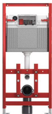
TECElux 100, Артикул 9600100
