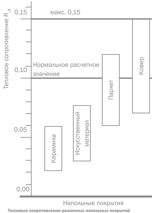
Тепловые сопротивления различных напольных покрытий
