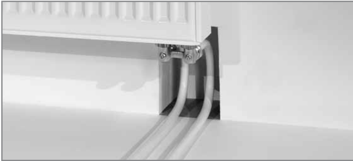
Подключение радиатора из стены
