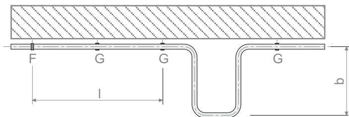
b — длина компенсатора, мм; l — длина трубы, м; F — неподвижная опора; G — скользящая опора.
