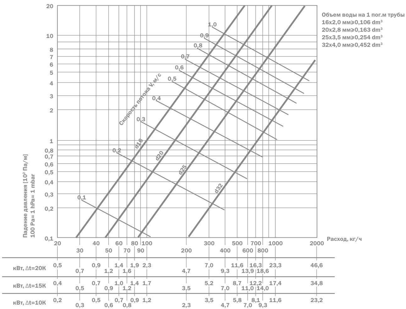
Диаграмма падения давления для универсальных многослойных труб в системах отопления
