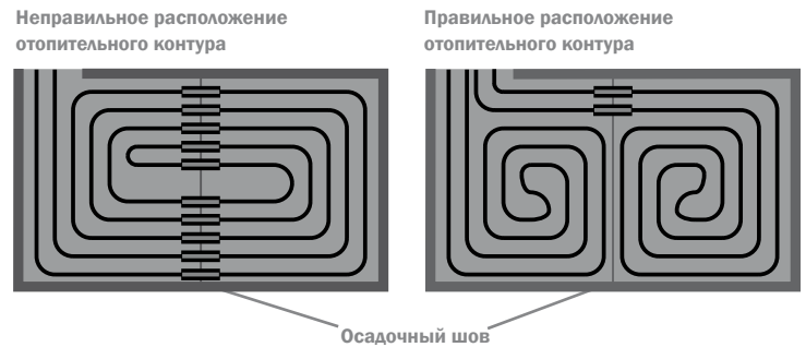
Схема укладки трубопровода при наличии расширительных швов
