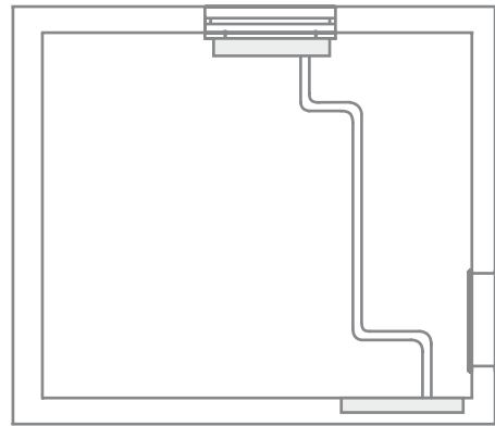
Пример прокладки трубопровода от распределителя к радиатору
