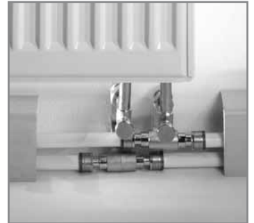
Подключение радиатора с использованием двойного тройника при плитусной проводке
